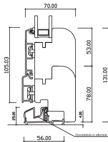
SEZIONE VERTICALE NODO INFERIORE PORTAFINESTRA MOD.STANDARD
