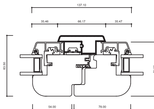
SEZIONE ORIZZONTALE FINESTRA E PORTAFINESTRA NODO CHIUSURA CENTRALE MOD.STANDARD
