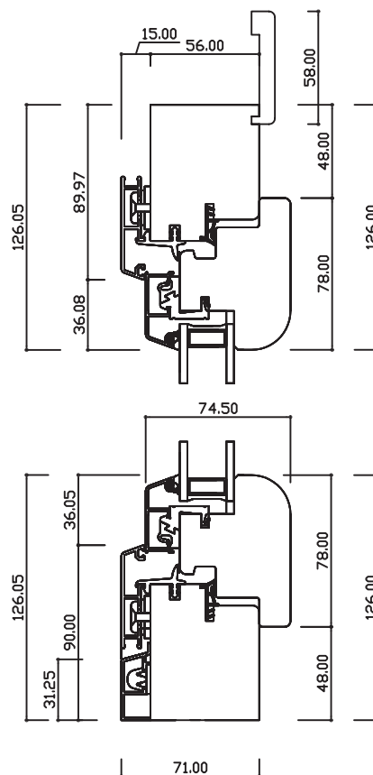
SEZIONE VERTICALE FINESTRA NODO INF.E SUP,TELAIO SISTEMA 5000/S MOD.STANDARD
